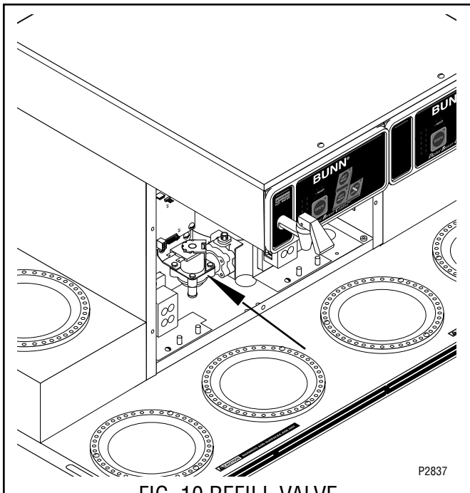
FIG. 10 REFILL VALVE
