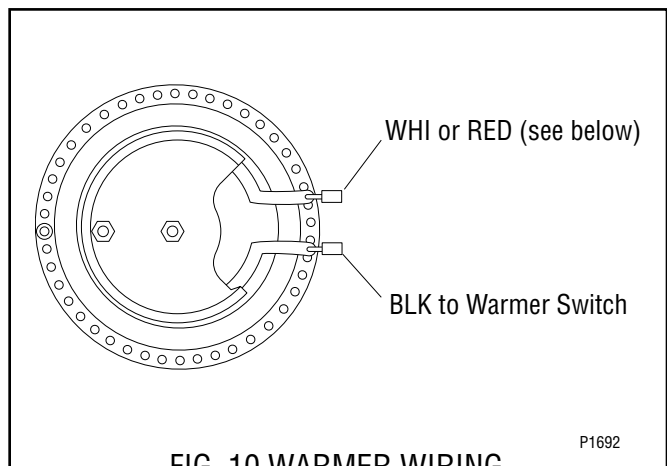
FIG. 10 WARMER WIRING
