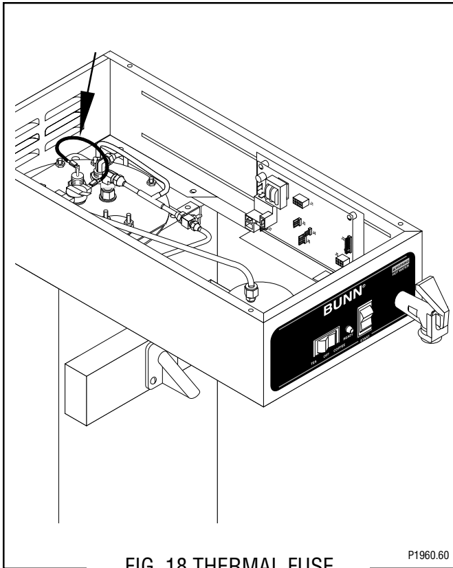
FIG. 18 THERMAL FUSE
