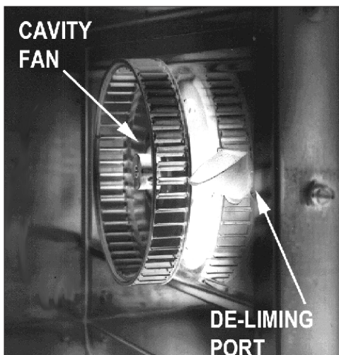
Cavity Fan
