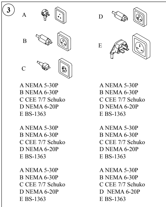
3 Plug Configurations Steckerkonfigurationen Configurations de prise
