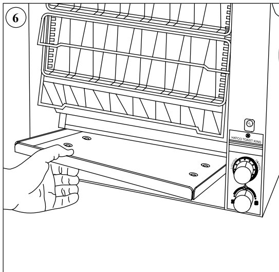
6 Install Toast Collector Pan Toast-Auffangbehälter installieren Installation du bac de récupération des toasts Toastverzamelpan installeren Instalar el recipiente para recoger las tostadas Installazione del vassoio di raccolta del pane
