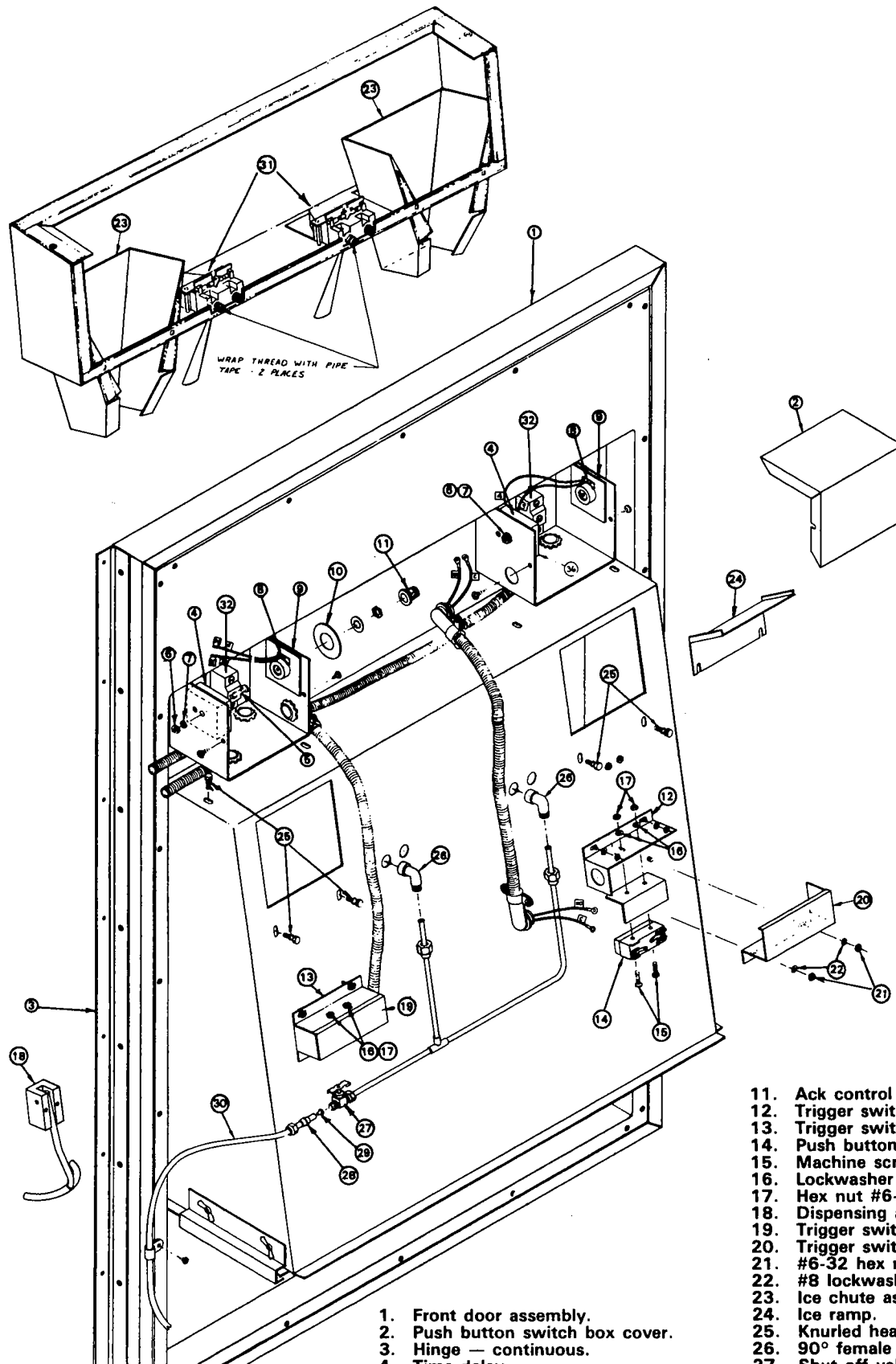
FIG. 19 AM-0654 DOOR COMPONENTS
