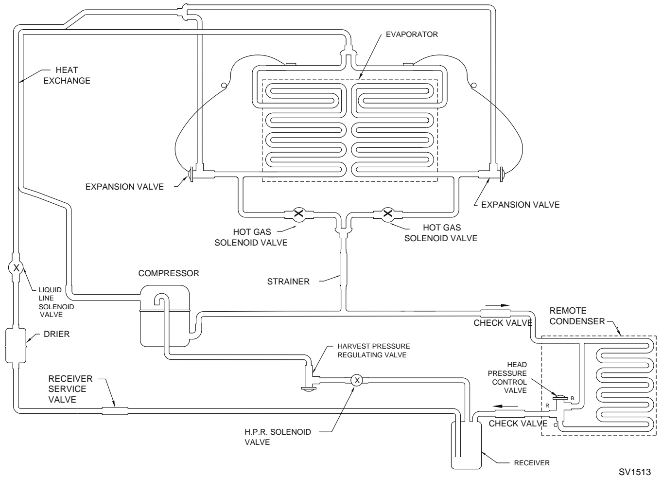
Figure 7-7. Q1300/Q1600/Q1800 Remote Models
