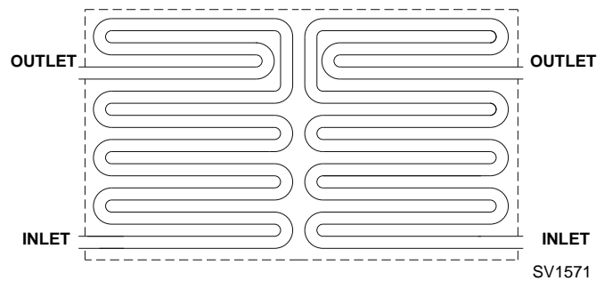
Figure 7-11. Q1300/Q1600/Q1800 Evaporator Tubing
