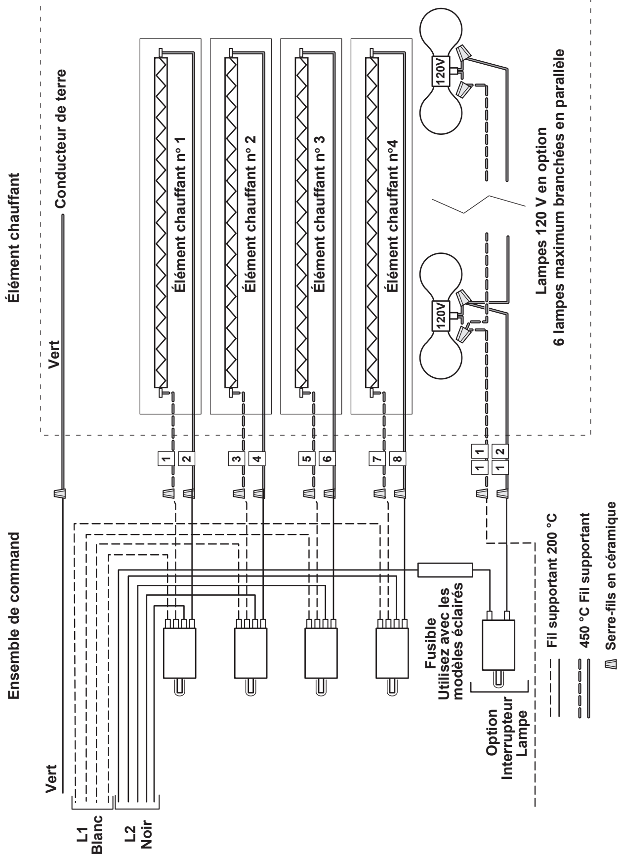
Diagramme de câblage de l'élément chauffant 208 - 240 V avec interrupteur à bascule
