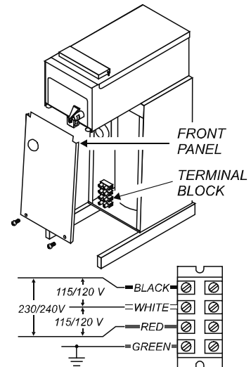
Fig. 3 115/230 Volt Terminal Block
