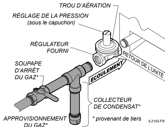
Fig. 2 Conduit d'approvisionnement du gaz
